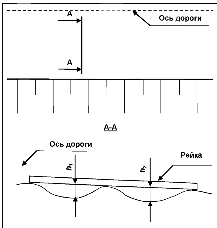
Рисунок 1 – Схема проведения измерений величины колеи
