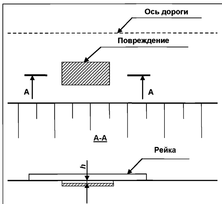
Рисунок 6 – Схема проведения измерений величины углубления ямочного ремонта
