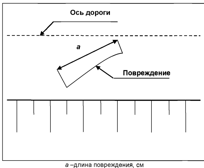
Рисунок 11 – Схема проведения измерений величины геометрических размеров трещины
